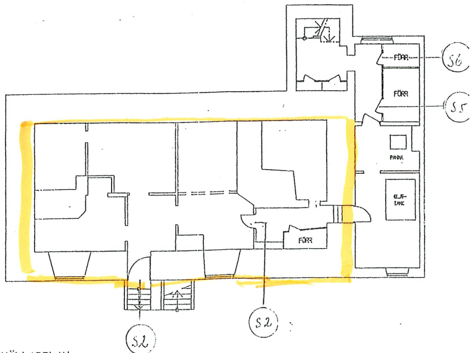
KÄLLARPLAN
